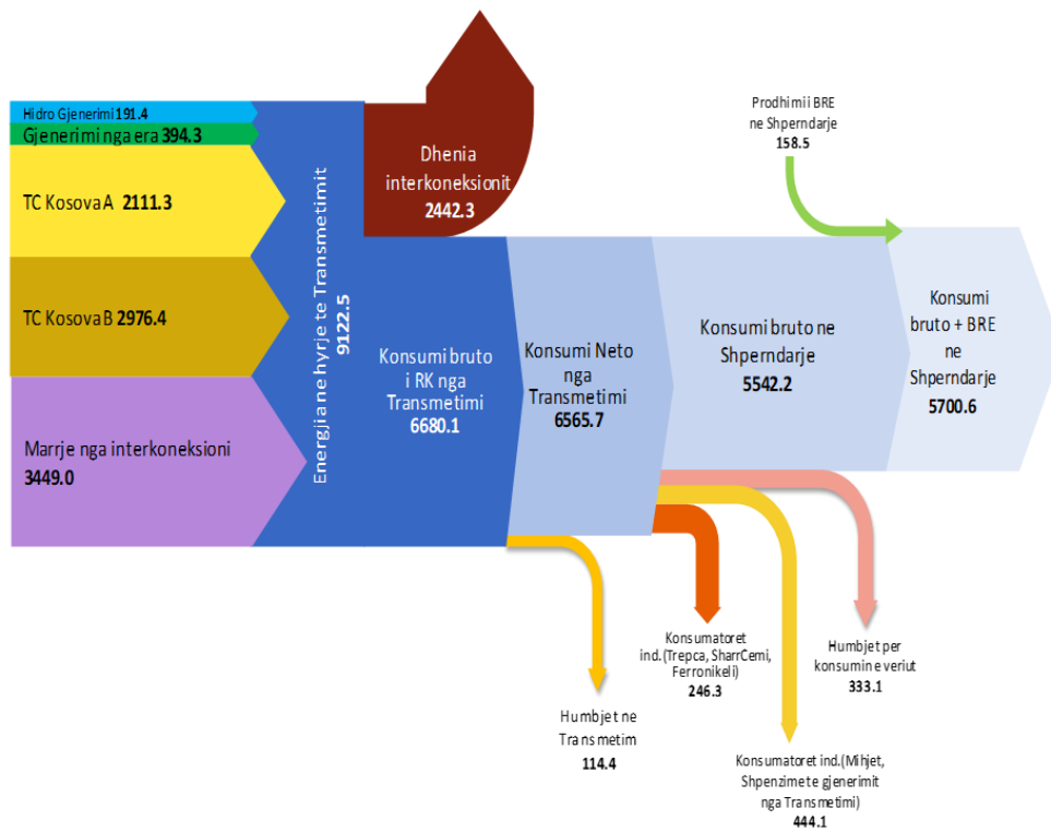
Figura 4. Bilanci i realizuar i energjisë elektrike në GWh janar-dhjetor 2023
