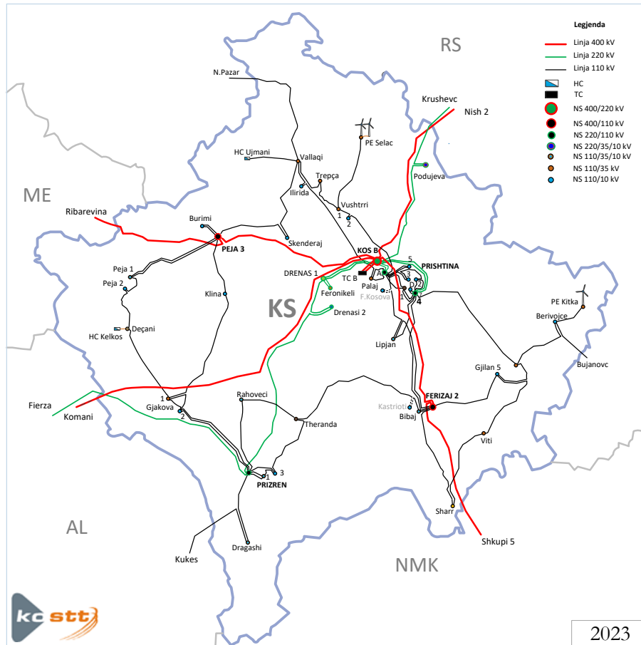
Figura 5. Shtrirja gjeografike e Sistemit Elektroenergjetik të Kosovës sipas gjendjes aktuale (2023).
